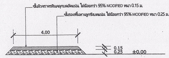
รูปตัดคั่นทาง กม. +0.036 ถึง +0.310
