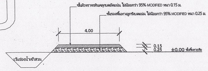
รูปตัดคั่นทาง กม. +0.000 ถึง +0.036
