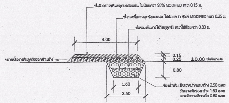
รูปตัดคั่นทาง กม. +0.036 ถึง +0.310
